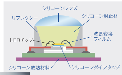
LEDの構造 (青字は当社の取り扱い製品)
