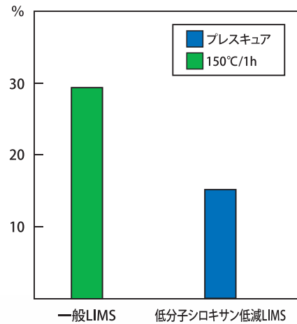
圧縮永久歪の比較データ
