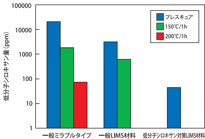
溶剤抽出法による低分子シロキサン量の比較データ
